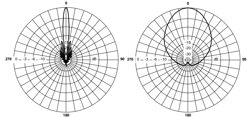
Диаграммы направленности антенны RFE 2400/60/18MIMO.
