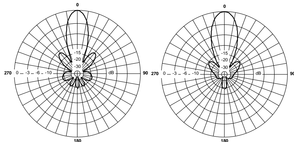
Диаграммы направленности антенны RFE 2300/16MBOX
