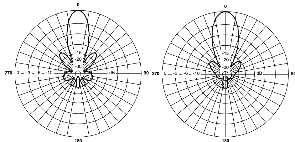
Диаграммы направленности антенны RFE 2400/16MBOX
