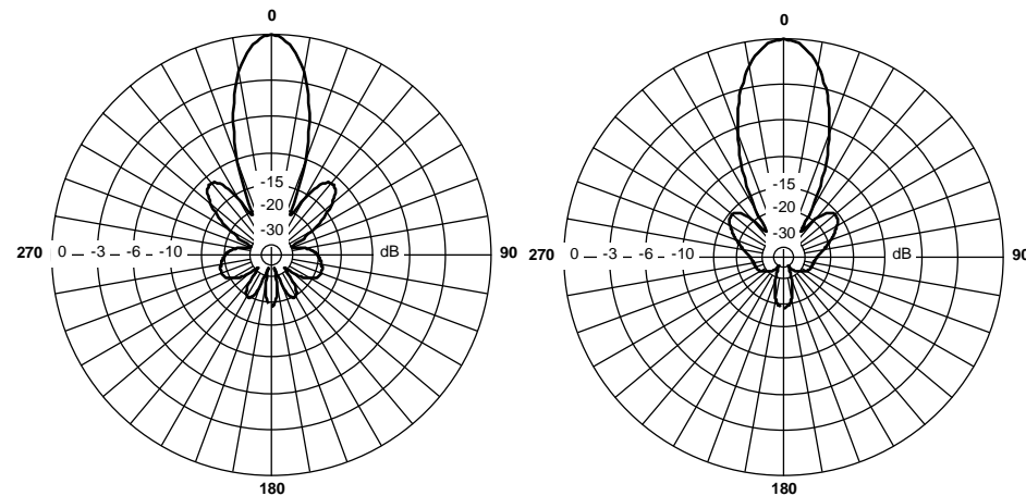
Диаграммы направленности антенны RFE 2700/16MBOX
