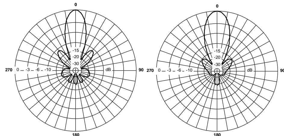
Диаграммы направленности антенны RFE 2300/16MIMO
